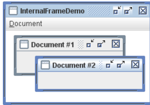
JInternalFrame
